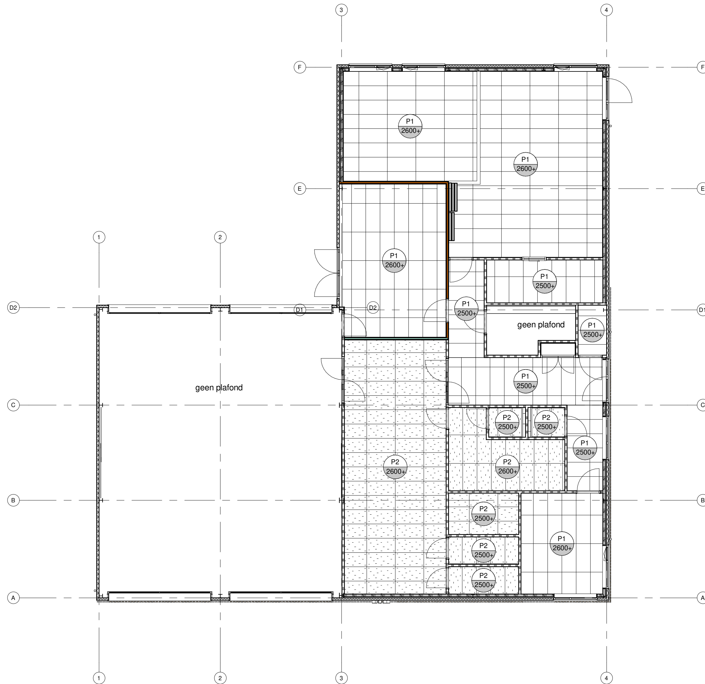
Plafond begane grond
