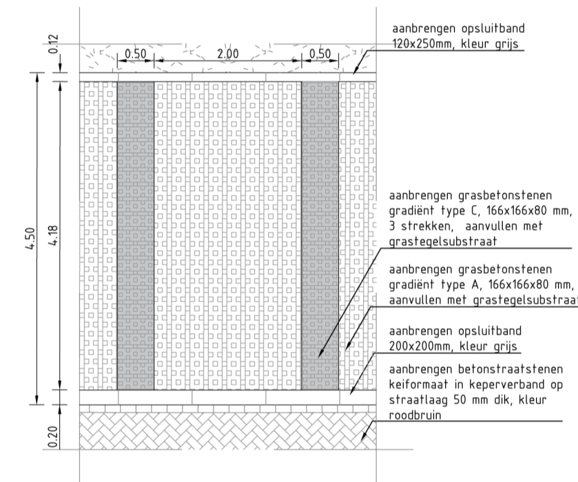
Detail haaksparkeren schaal 1:50
