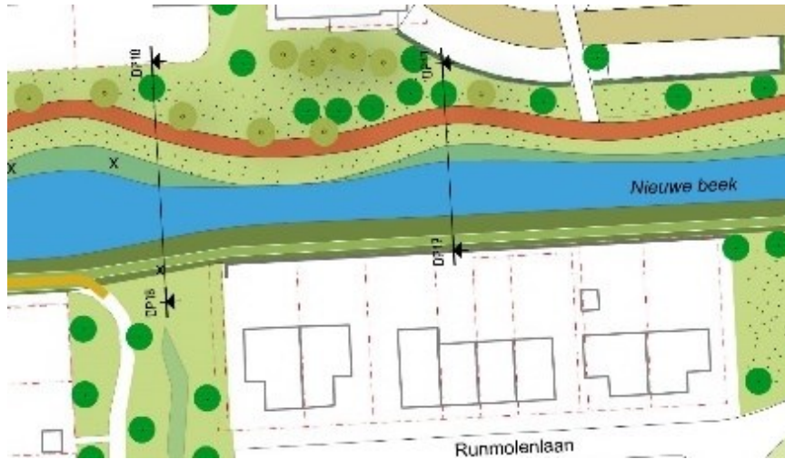
Nieuwe beek_profiel 17_huidige situatie
