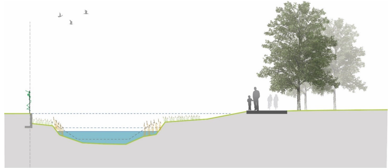
Nieuwe beek_profiel 17_huidige situatie
