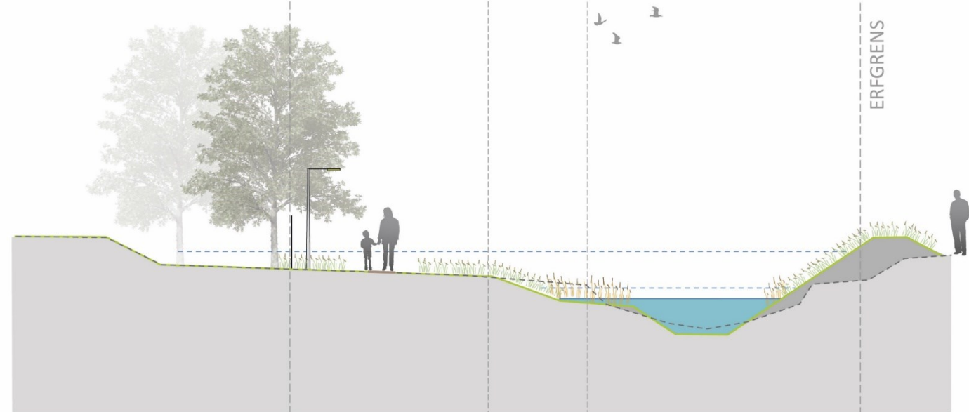
Barchemse Veengoot_profiel 9_principe legger
