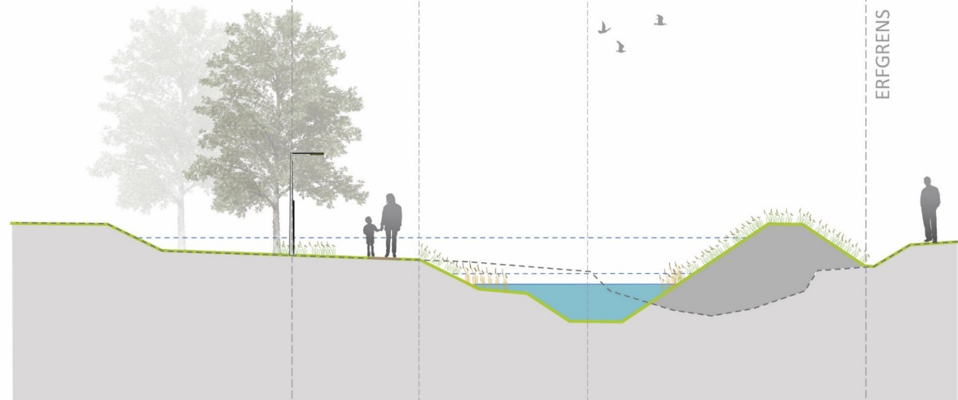
Barchemse Veengoot_profiel 9_principe erfgrens
