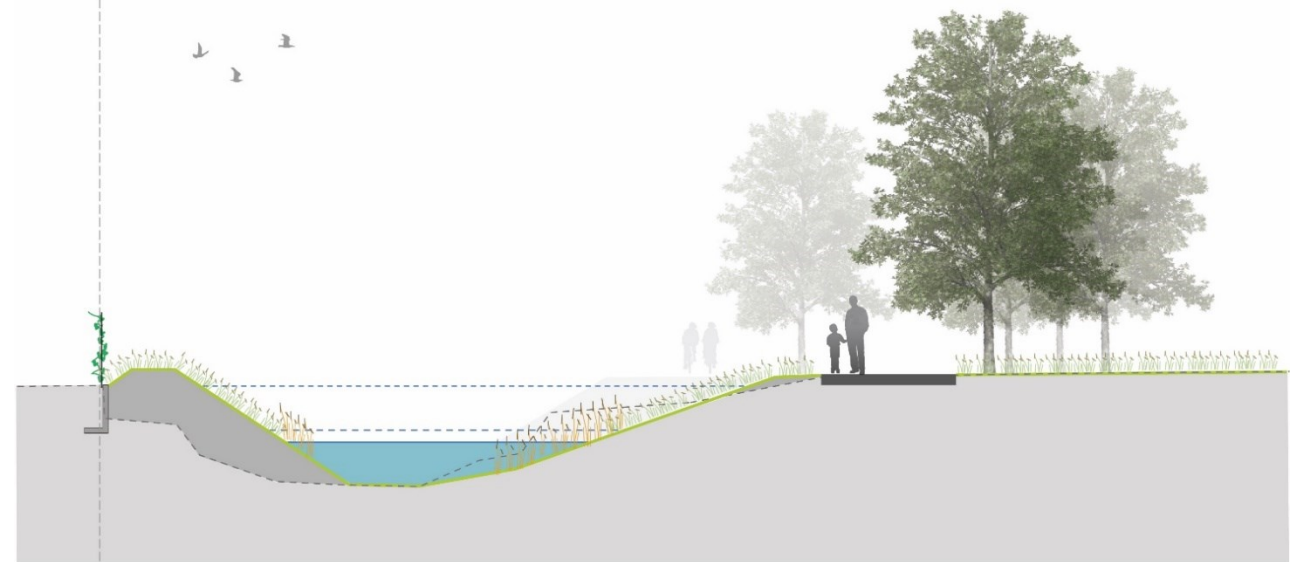
Nieuwe beek_profiel 17_schetsontwerp
