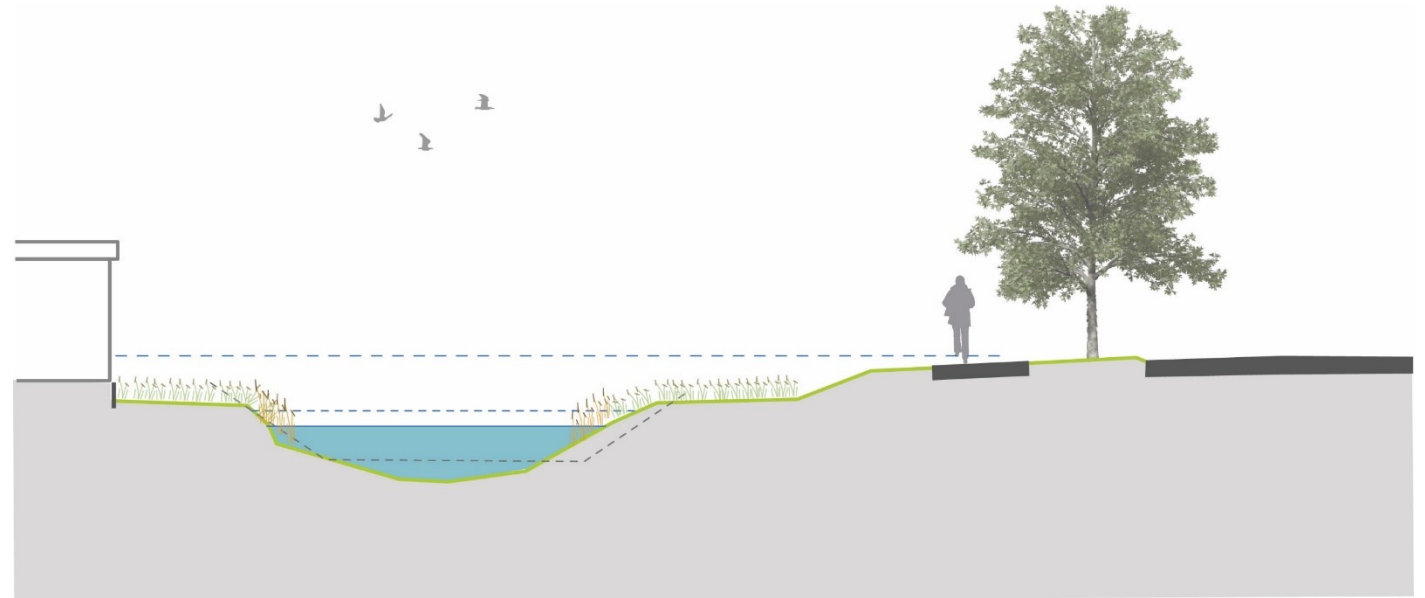
Nieuwe beek_profiel 22_huidige situatie
