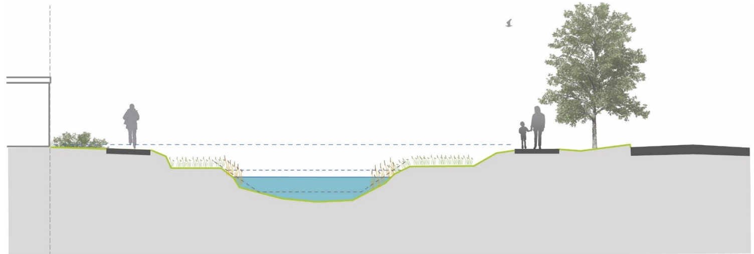
Nieuwe beek_profiel 20_huidige situatie
