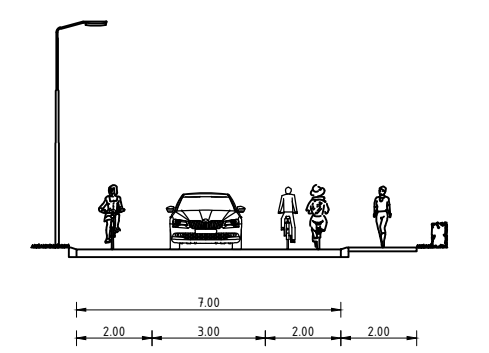
Dwarsdoorsnede B
