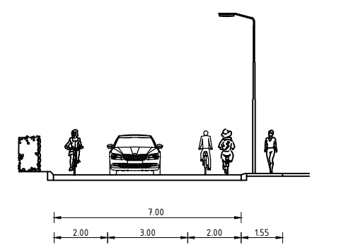
Dwarsdoorsnede A
