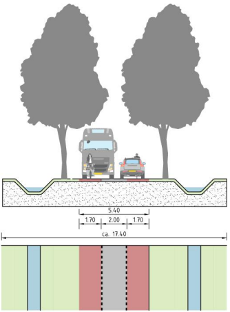
Doorsnede A-A Schaal 1:200
