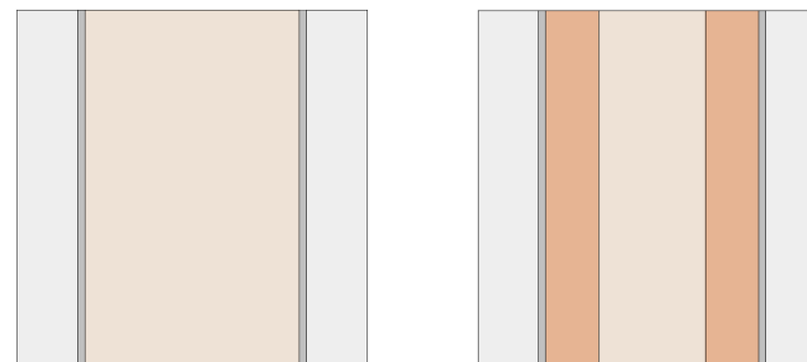
Figuur 37: ETW B met en zonder fietssuggestiestrook
